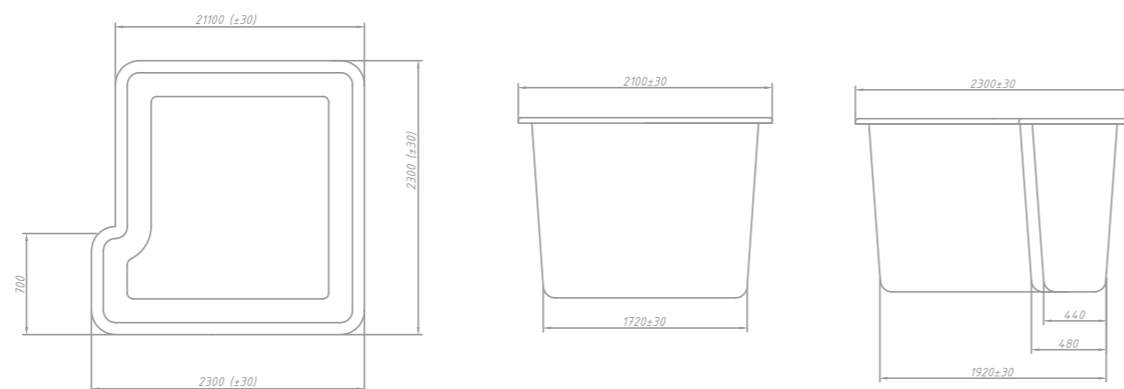
ГАБАРИТНЫЕ РАЗМЕРЫ
