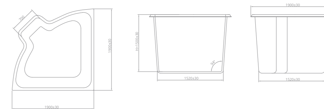
ГАБАРИТНЫЕ РАЗМЕРЫ
