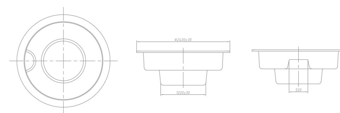
ГАБАРИТНЫЕ РАЗМЕРЫ
